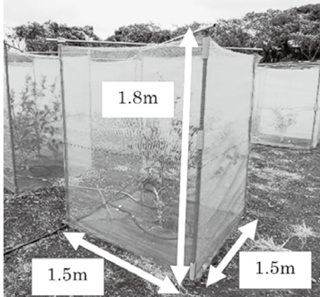
写真1 簡易防風ユニット構造
